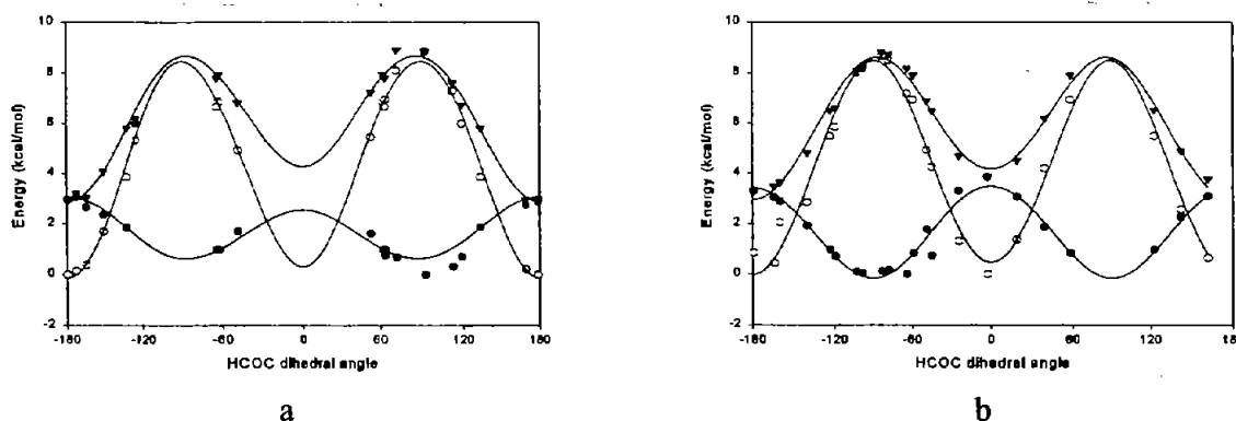
Figura 2.13. Dependencia de la energía de deleción de las interacciones n_p \rightarrow \sigma^*_{\text{C-H}} (○), n_s \rightarrow \sigma^*_{\text{C-H}} (●) y n_s + n_p \rightarrow \sigma^*_{\text{C-H}} (▼) en relación con el ángulo diedro HCOC en: a) oxano, b) etil-metil-éter.
