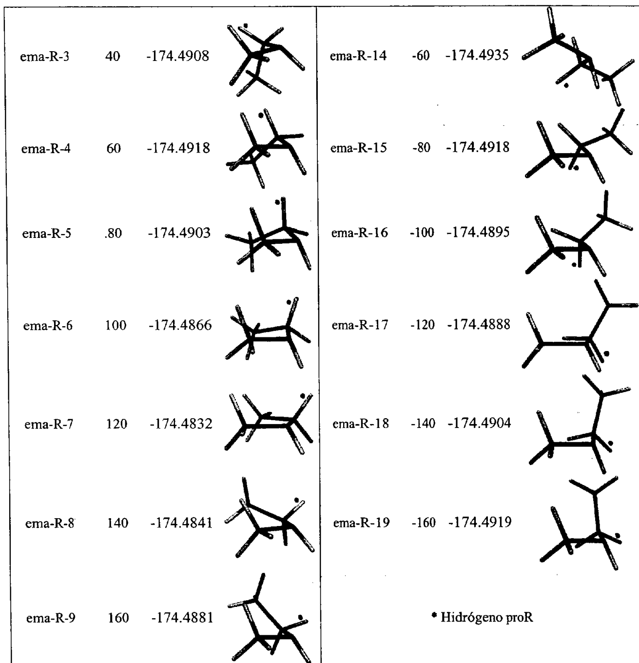
Figura 2.34. Conformeros de la (R)-ema restringida en el ángulo diedro H_{\text{proR}}\text{-C-N-C} .
