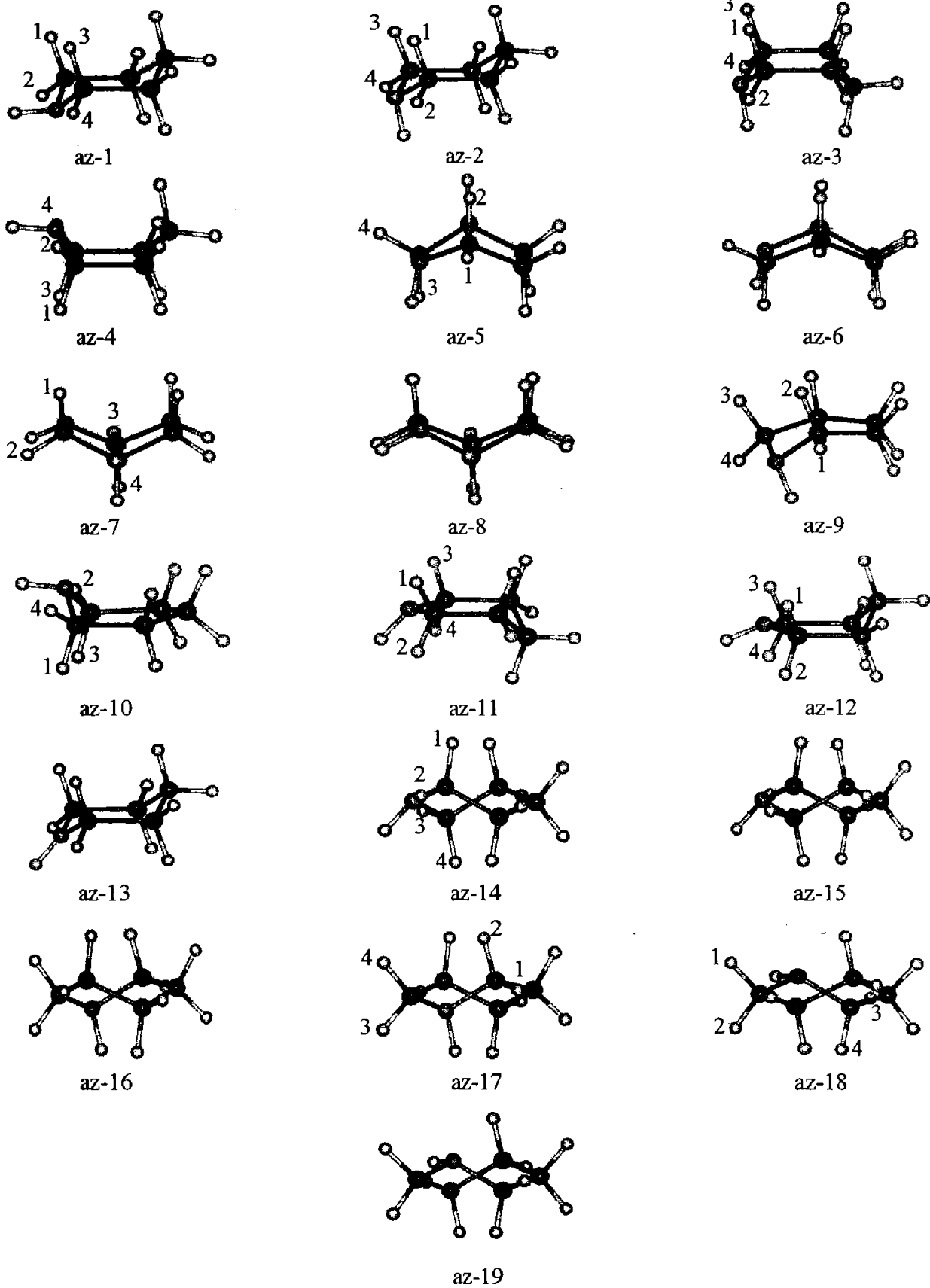
Figura 2.29. Conforméros del azano presentes en su proceso de inversión.
