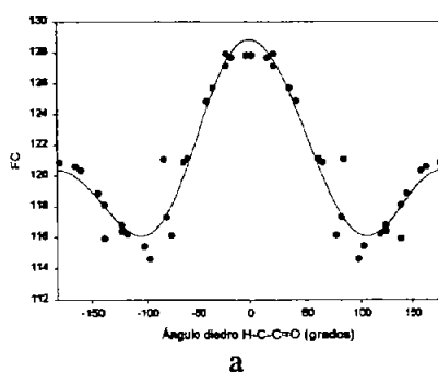
Figura 2.38. Variación del contacto de Fermi respecto al giro de la etil-metil-cetona
