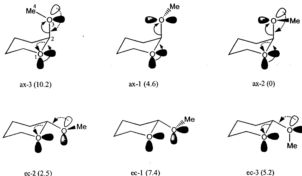
Figura 4.7. Interacciones endo -anoméricas ( \rightarrow ) y exo -anoméricas ( \cdots\rightarrow ). En paréntesis, la energía total corregida en kcal/mol calculada con MP2 después de sustraer E_{ax-2} a partir de cada valor de E.
