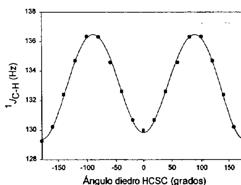
Figura 2.28. Constante de acoplamiento ^1J_{C-H} (Hz) contra el ángulo diedro HCSC (grados) para los conformeros del dimetil-tioéter.
