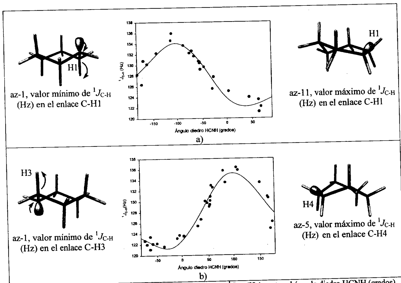
Figura 2.30. Dependencia de la constante de acoplamiento ^1J_{C-H} (Hz) contra el ángulo diedro HCNH (grados) para los conformeros del azano a) Grupo 1 y b) Grupo 2.
