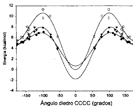
Figura 2.41 Dependencia de la Energía de deslocalización \sigma_{\text{C-H}} \rightarrow \pi^*_{\text{C=O}} en: (•) etil-metil-cetona, (o)etil-metil-tiocetona y (▼) 2-metilbuteno.
