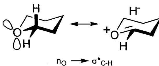
Figura 2.5. Híbrido de doble enlace-no enlace
