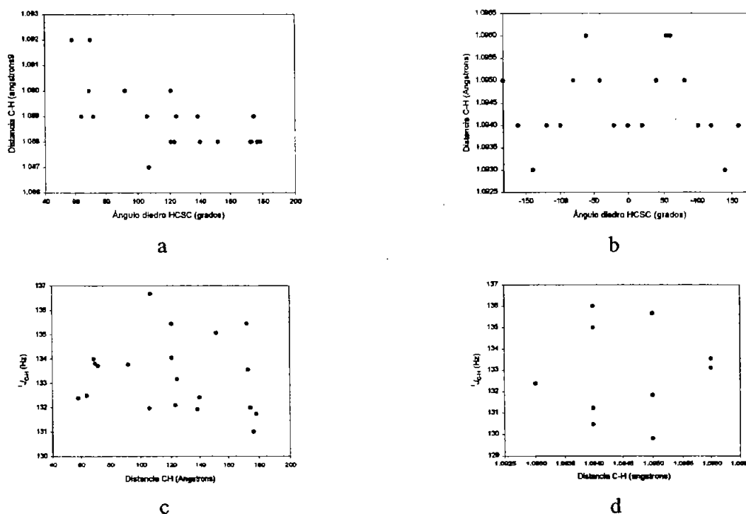
Figura 2.27. Distancia C-H en función del ángulo diedro HCSC. a) tiano, b) emte. ^1J_{CH} en función de la distancia C-H c) tiano, d) emte.
