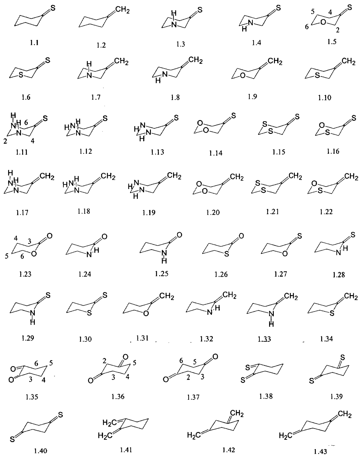
Figura 1.6 Moléculas estudiadas
