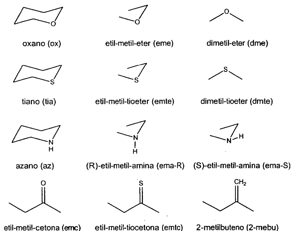
Figura 2.6. Moléculas estudiadas
