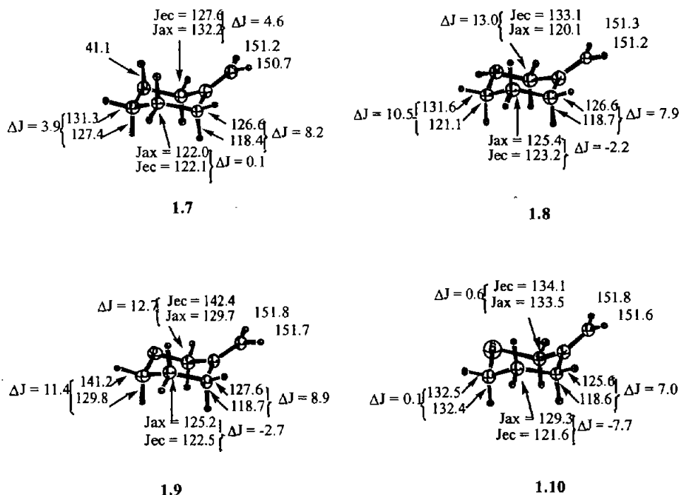
Figura 1.10. Constantes de acoplamiento C-H (Hz) en hetero-metilciclohexanos.
