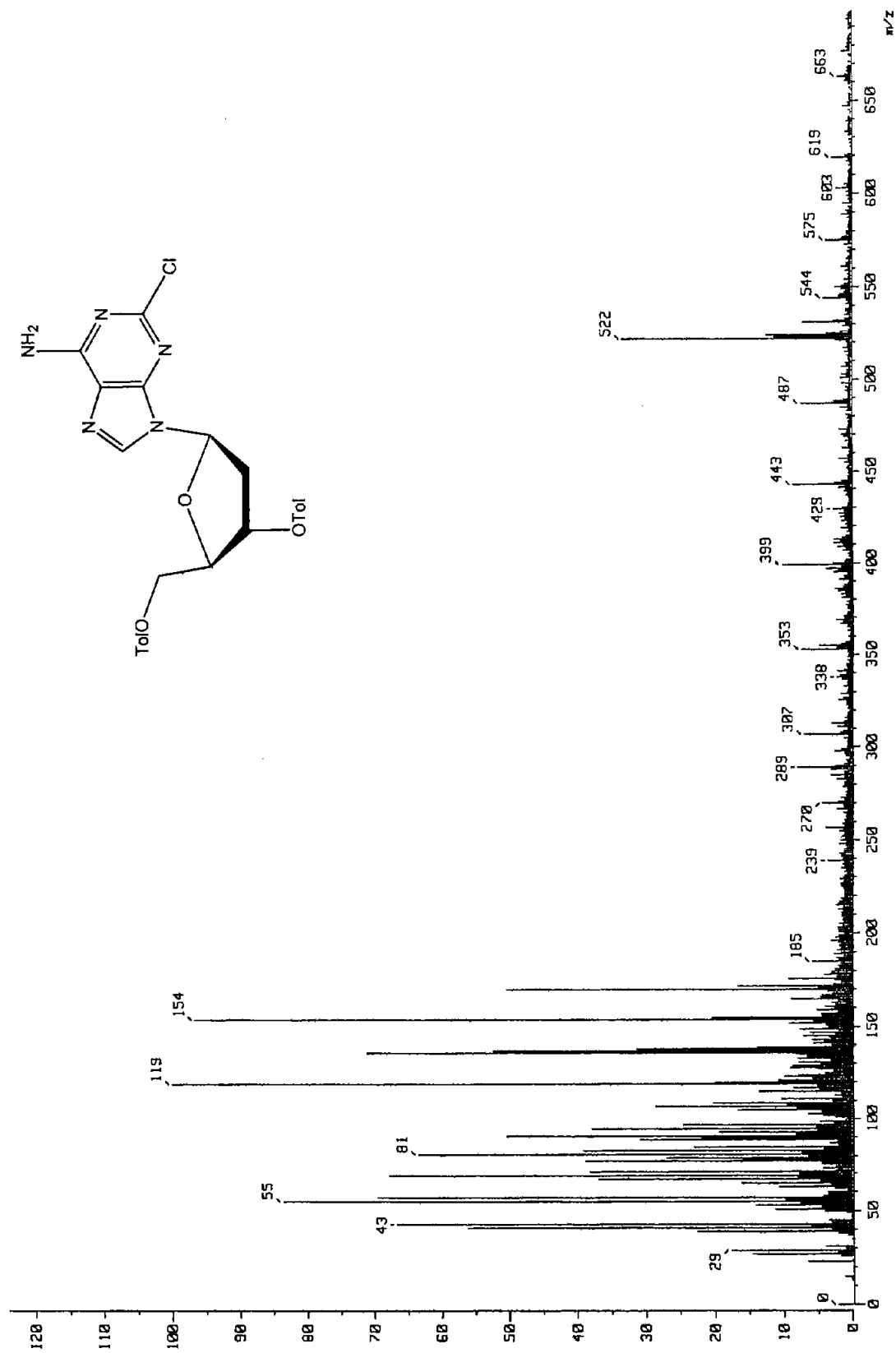
83 Espectro 16. EM (FAB + ) de 2-cloro-6-amino-9-(2'-desoxi-3', 5'-di-O-p-toluid-β-D-eritro-pentofuranosil)purina (41).
