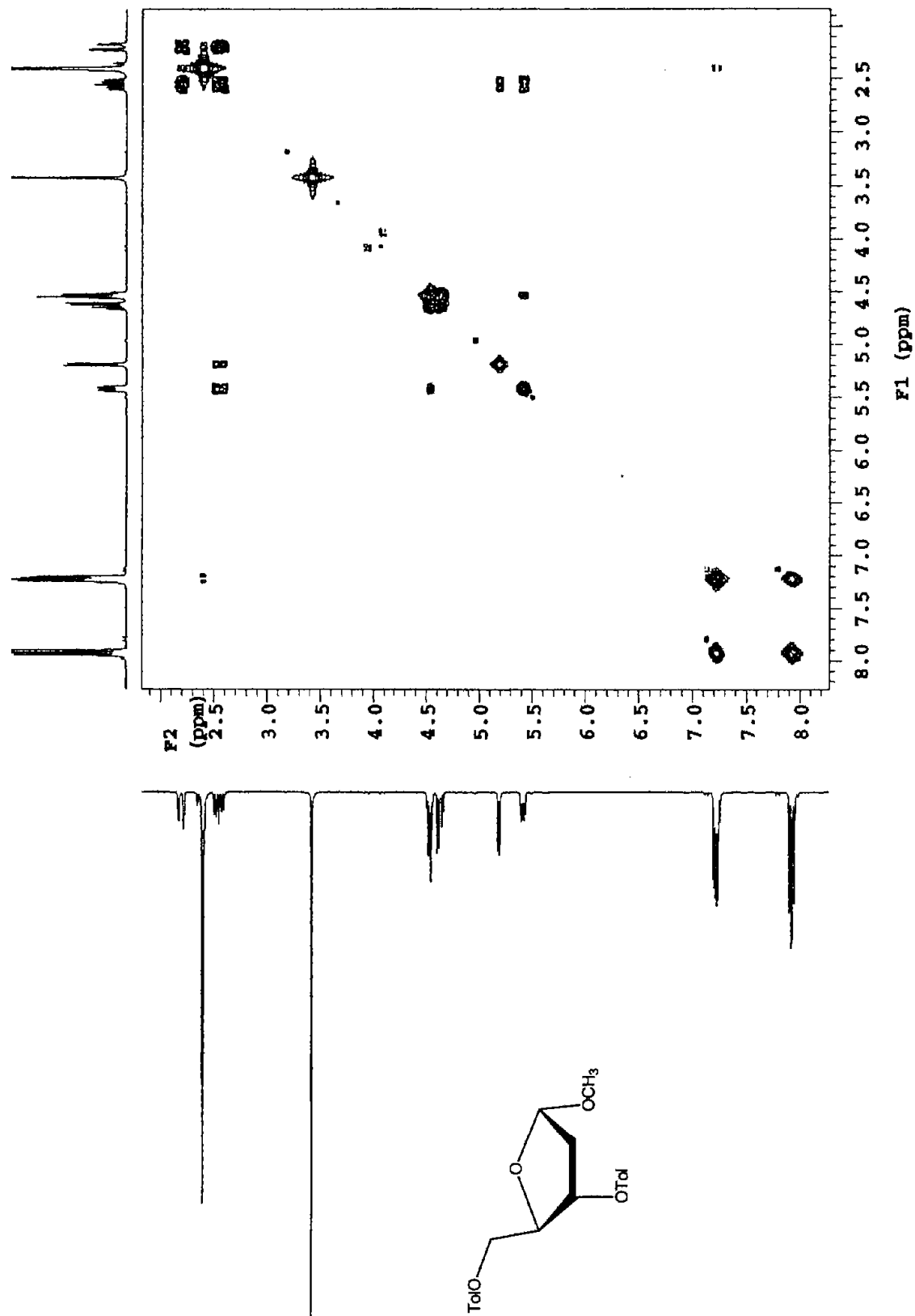
Espectro 3. COSY (300 MHz, CDCl 3 ) de 2-desoxi-3,5-di-O- p -toluid- \alpha -D-eritro-pentofuranósido de metilo (12a).
