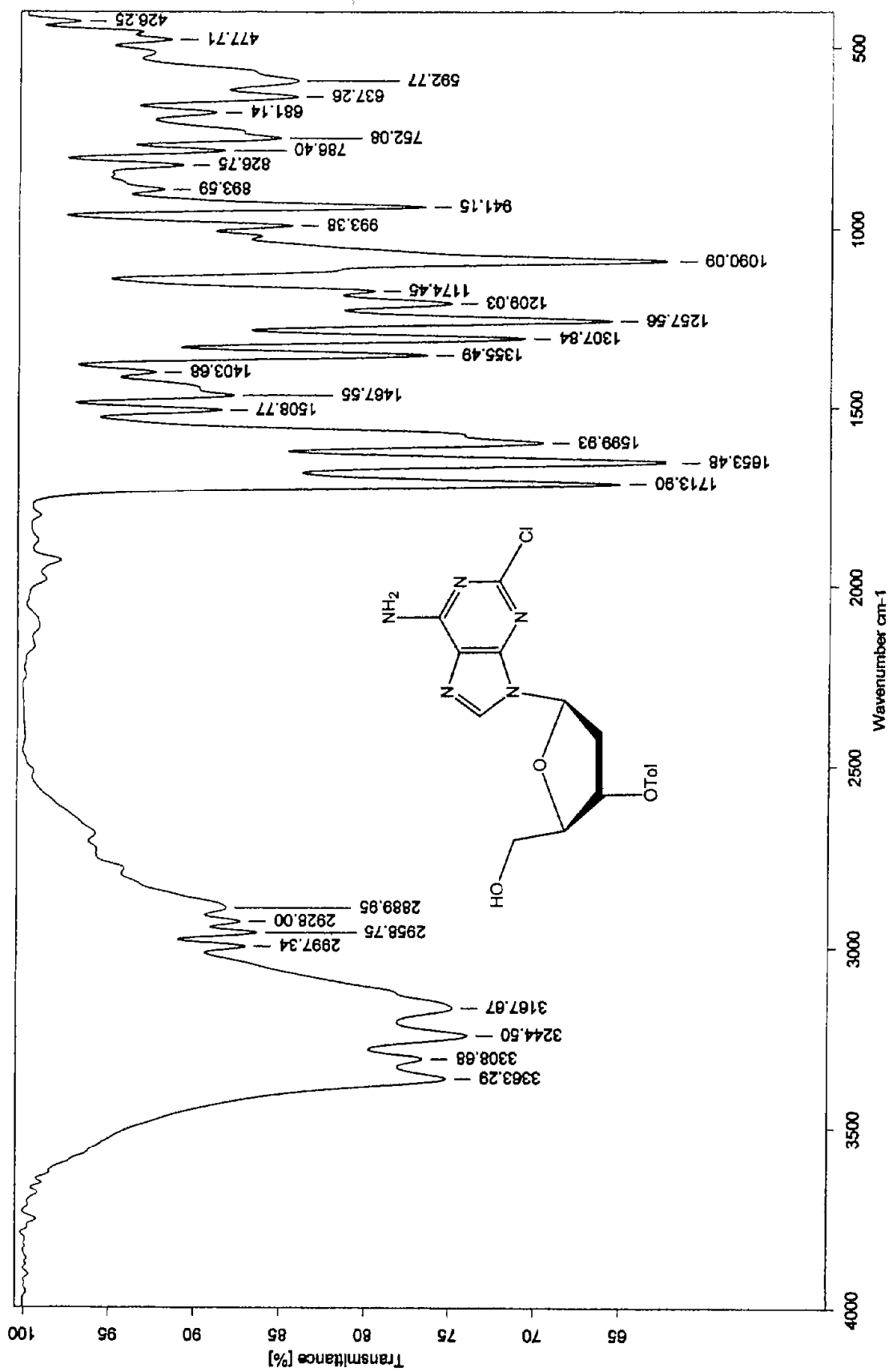
Espectro 20. IR (KBr) de 2-cloro-6-amino-9-(2'-deoxi-3'-O-p-toluid-β-D-eritro-pentofuranosil)purina (42).
