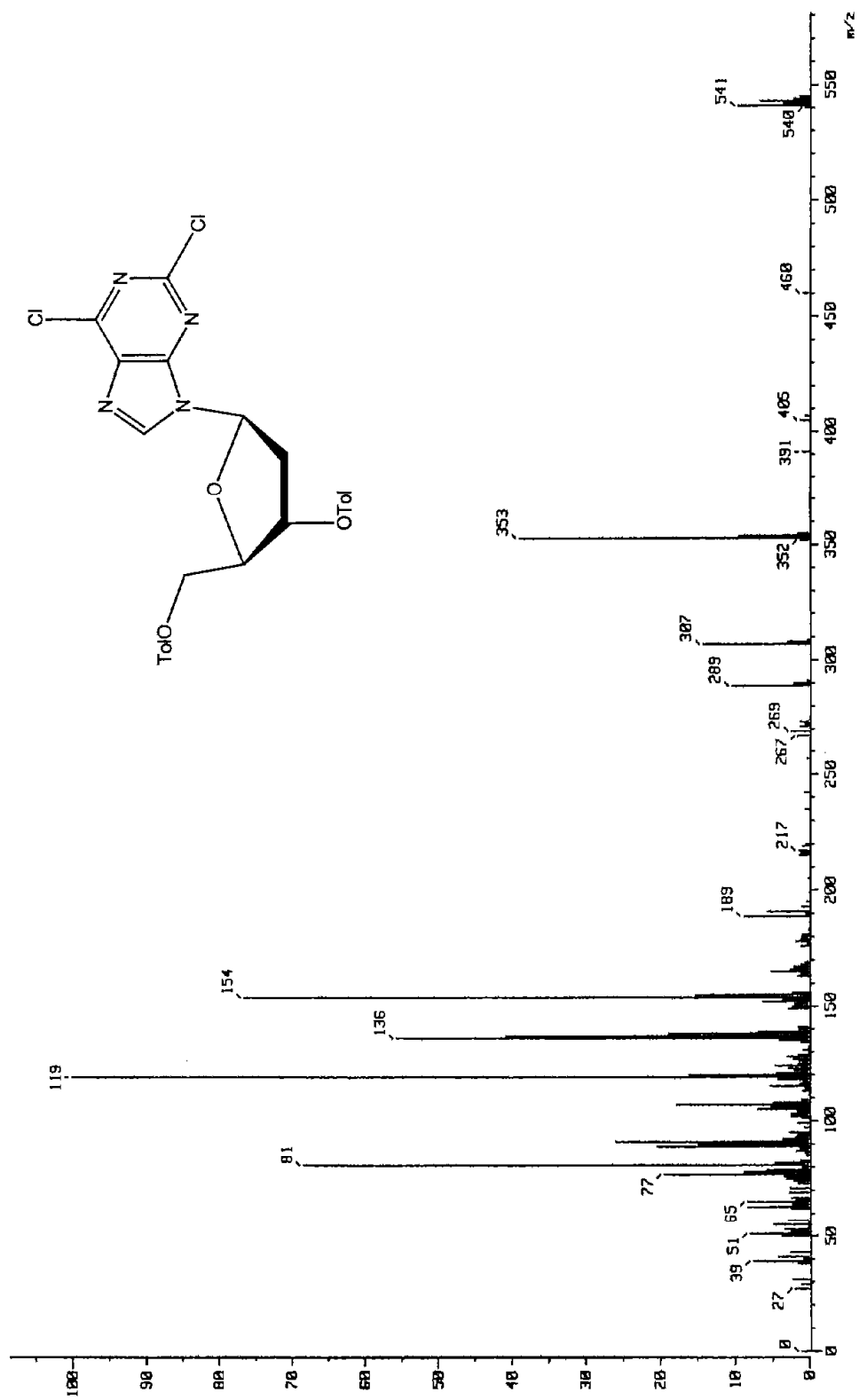
Espectro 13. EM (FAB + ) de 2,6-dicloro-9-(2'-desoxi-3', 5'-di-O-p-toluid-β-D-eritro-pentofuranosil)purina (28a).
