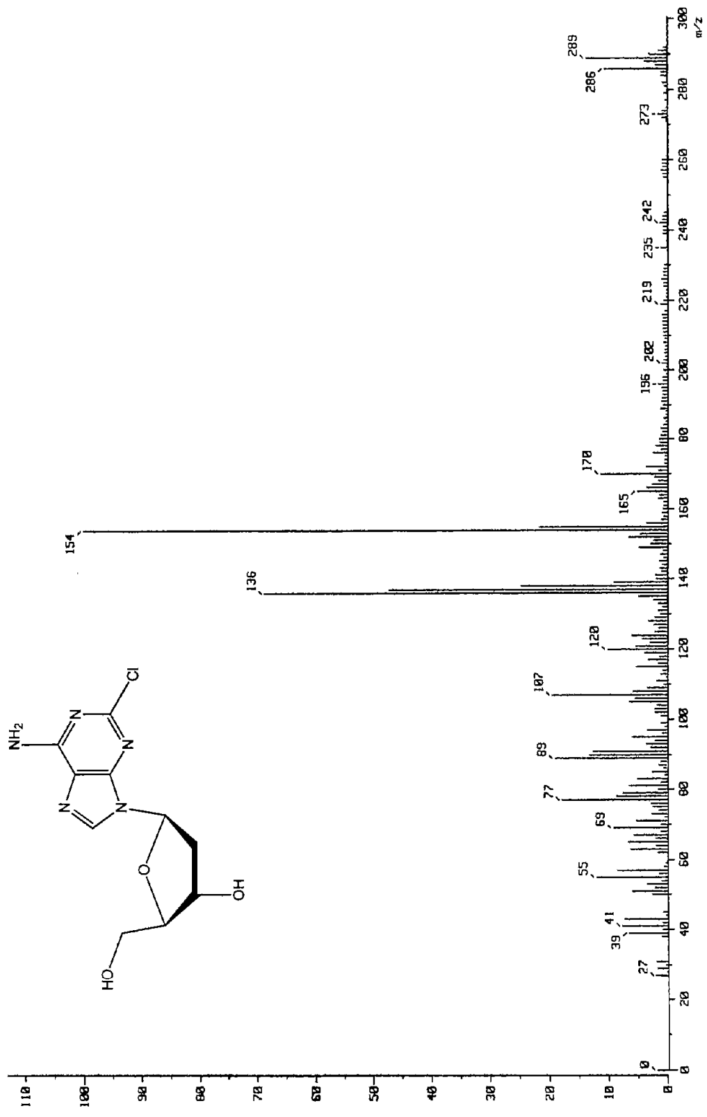
Espectro 26. EM (FAB + ) de 2-cloro-6-amino-9-(2'-desoxi-β-D-eritro-pentofuranosil)purina (35).
