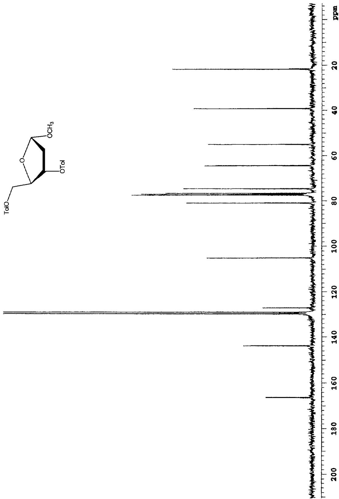
Espectro 2. RMN ^{13}\text{C} (75 MHz, \text{CDCl}_3 ) de 2-desoxi-3,5-di-O-p-toluid- \alpha -D-eritro-pentofuranósido de metilo (12a).
