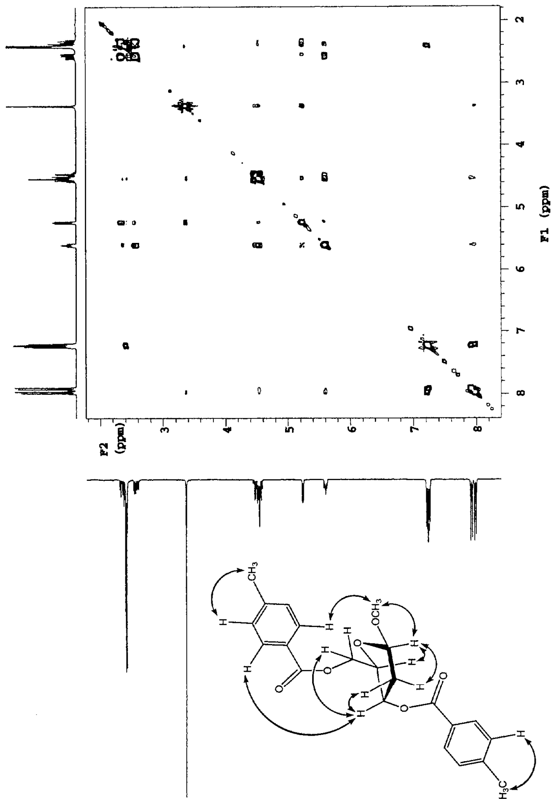
Espectro 10. NOESY (300 MHz, CDCl 3 ) de 2-desoxi-3,5-di-O- p -toluid-β-D-eritro-pentofuranosido de metilo (12b).
