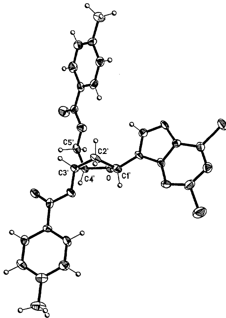
Figura 8. Estructura molecular para la 2,6-dicloro-9-(2'-desoxi-3', 5'-di-O- p -toluid-β-D- eritro -pentofuranosil)purina (28a).
