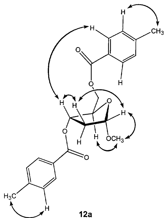
Figura 3. Interacciones NOESY relevantes de 2-desoxi-3,5-di-O- p -toluidl- \alpha -D-eritro-pentofuranósido de metilo (12a).
