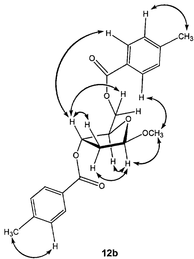
Figura 4. Interacciones NOESY relevantes de 2-desoxi-3,5-di-O- p -toluid-β-D-eritro-pentofuranósido de metilo ( 12b ).
