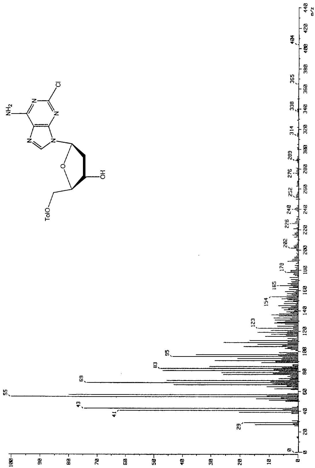
Espectro 22. EM (FAB + ) de 2-cloro-6-amino-9-(2'-desoxi-5'-O-p-toluidil-β-D-eritro-pentofuranosil)purina (43).
