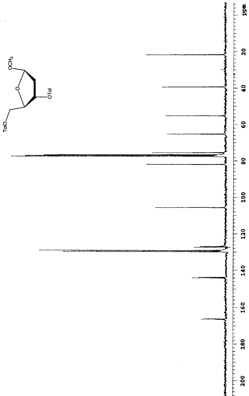
Espectro 8. RMN 13 C (75 MHz, CDCl 3 ) de 2-desoxi-3,5-di-O-p-toluid-β-D-eritro-pentofuranósido de metilo (12b).
