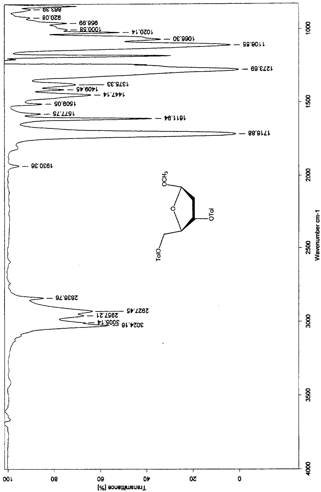
Espectro 12. IR (CHCl 3 ) de 2-deoxi-3,5-di-O-p-toluid-β-D-eritro-pentofuranosido de metilo (12b).
