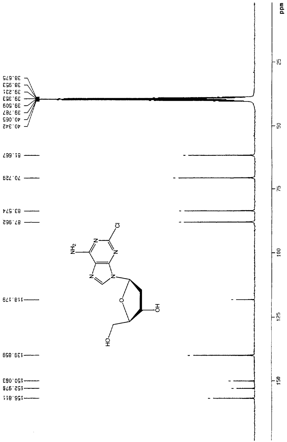
Espectro 25. RMN 13 C (75 MHz, DMSO-d 6 ) de 2-cloro-6-amino-9-(2'-deoxi-β-D-eritro-pentofuranosil)purina (35).
