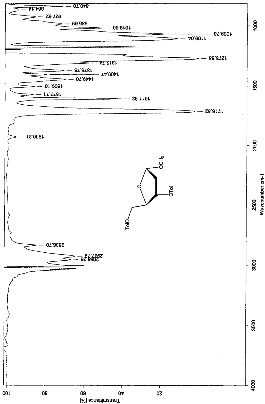
Espectro 6. IR (CHCl 3 ) de 2-desoxi-3,5-di-O-p-toluid- \alpha -D-eritro-pentofuranosido de metilo (12a).
