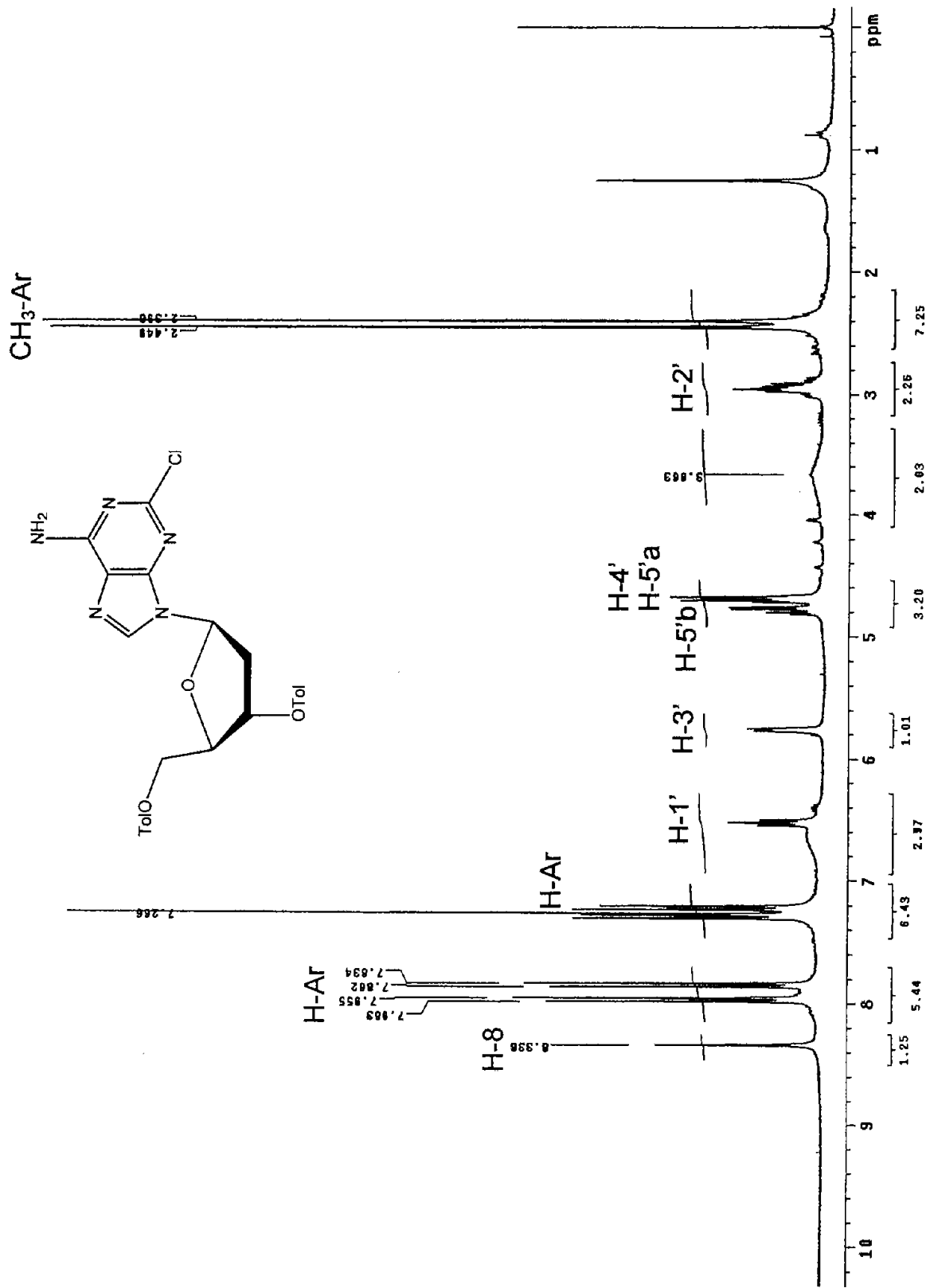
82 Espectro 15. RMN 1 H (300 MHz, CDCl 3 ) de 2-cloro-6-amino-9-(2'-desoxi-3', 5'-di-O-p-toluidl- \beta -D-eritro-pentofuranosil)purina (41)
