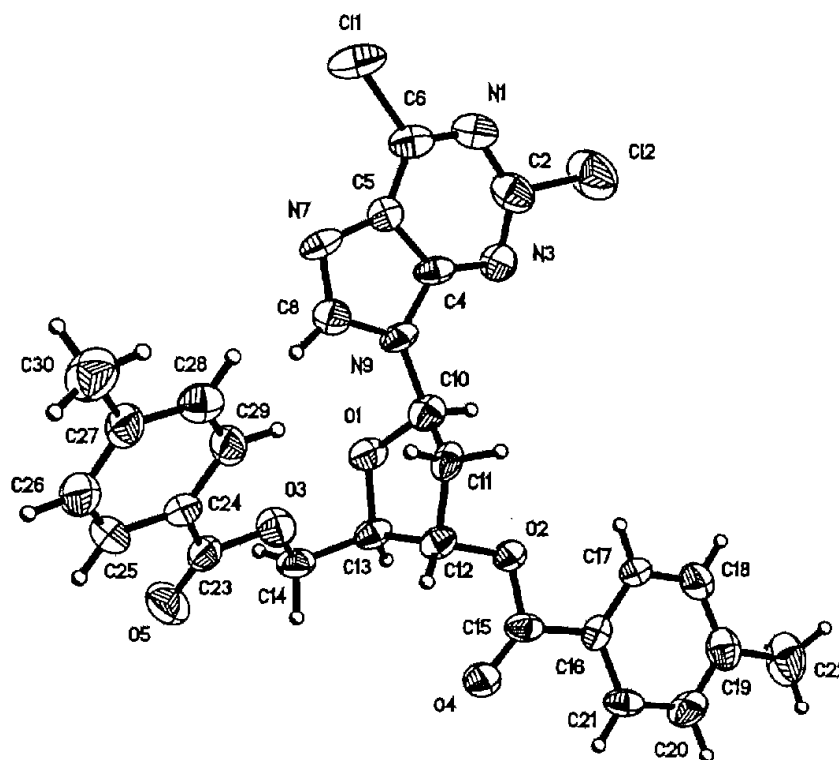
Figura 7. Estructura molecular para la 2,6-dicloro-9-(2'-desoxi-3', 5'-di-O- p -toluidil- \beta -D- eritro -pentofuranosil)purina ( 28a ).
