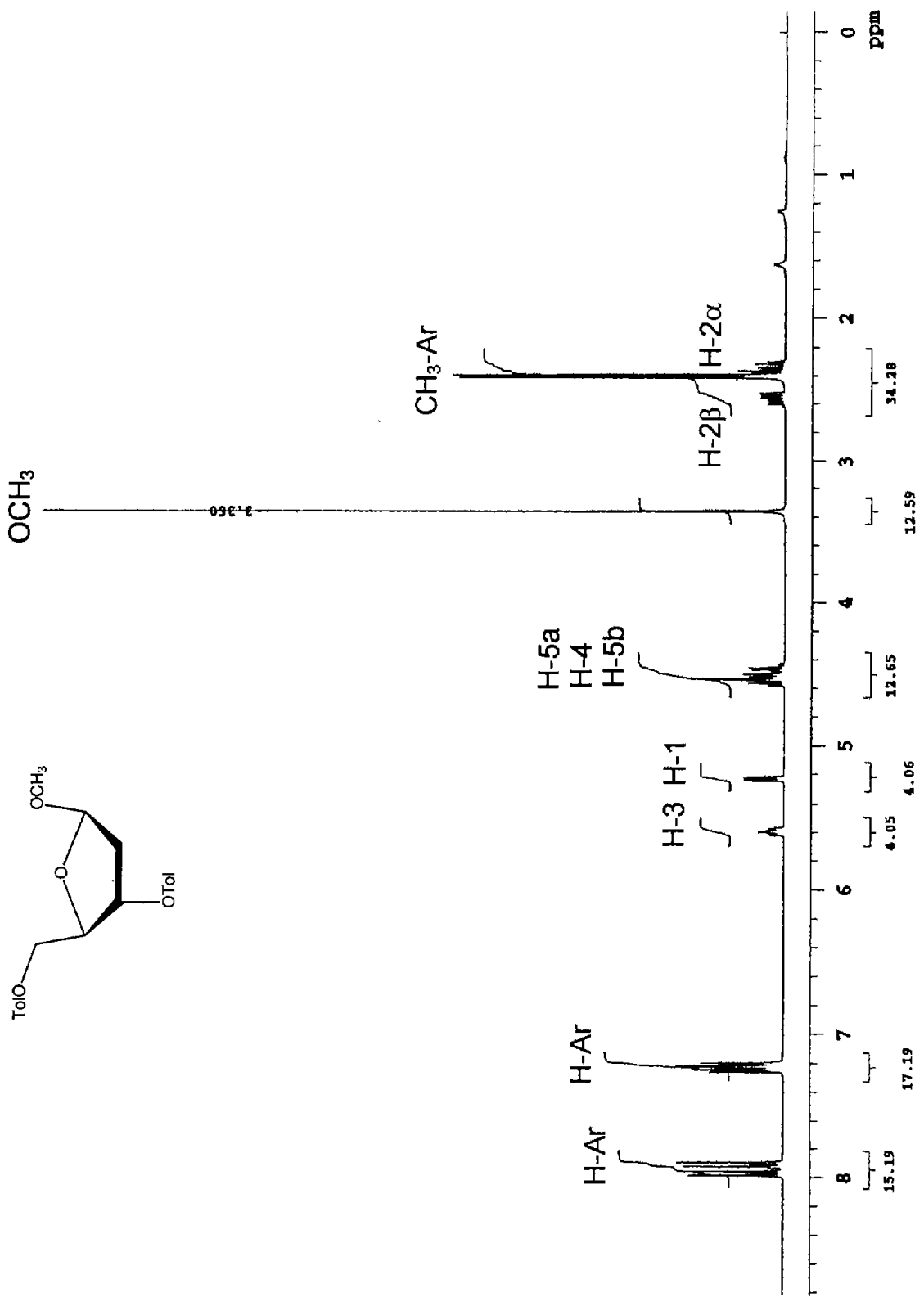
Espectro 7. RMN 1 H (300 MHz, CDCl 3 ) de 2-desoxi-3,5-di-O-p-toluidl-β-D-eritro-pentofuranósido de metilo (12b).
