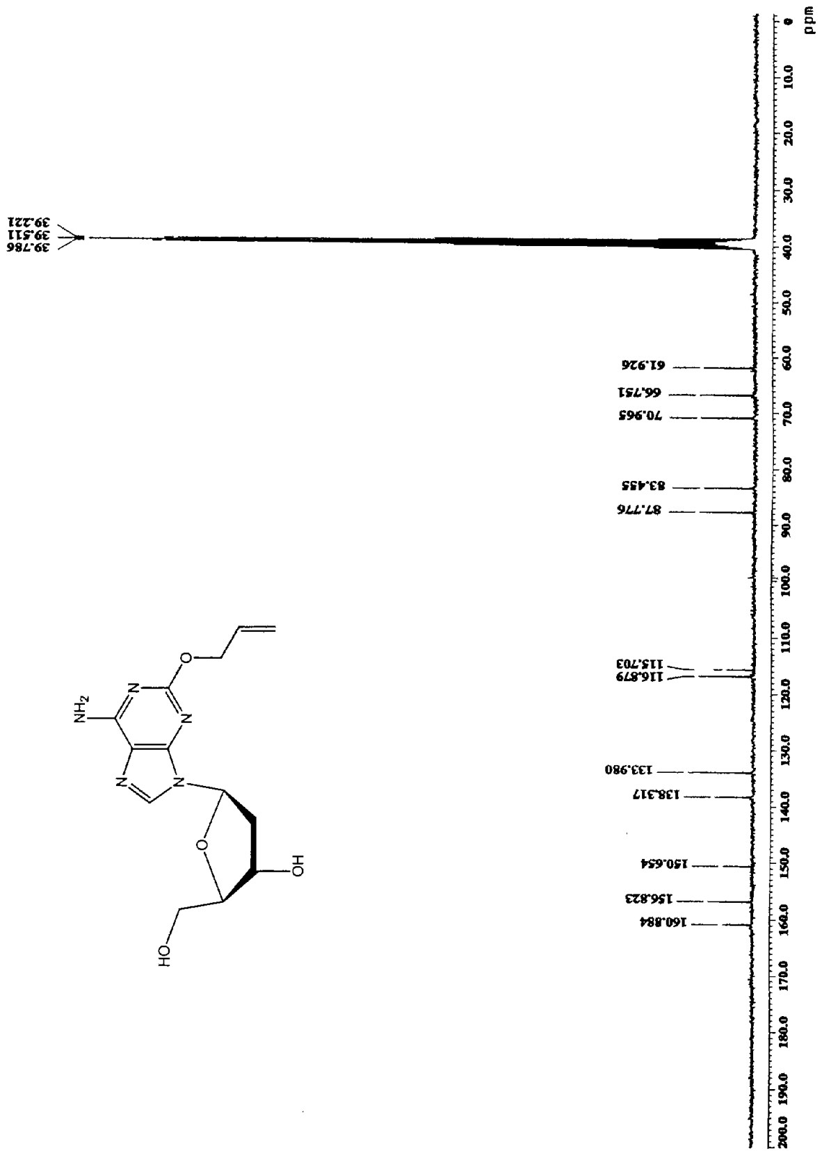
Espectro 29. RMN 13 C (75 MHz, DMSO-d 6 ) de 2-alioksi-6-amino-9-(2'-desoxi-β-D-eritro-pentofuranosil)purina (36).
