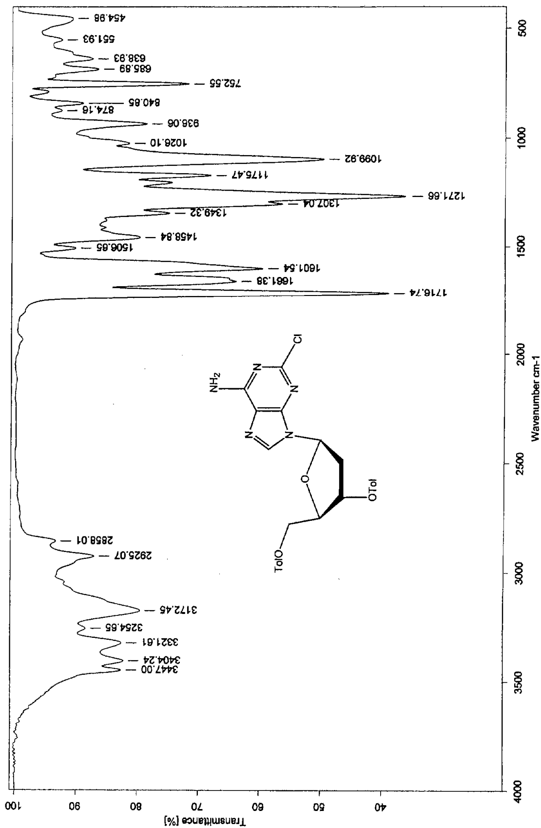
Espectro 17. IR (KBr) de 2-cloro-6-amino-9-(2'-deoxi-3', 5'-di-O-p-toluil-β-D-eritro-pentofuranosil)purina (41).
