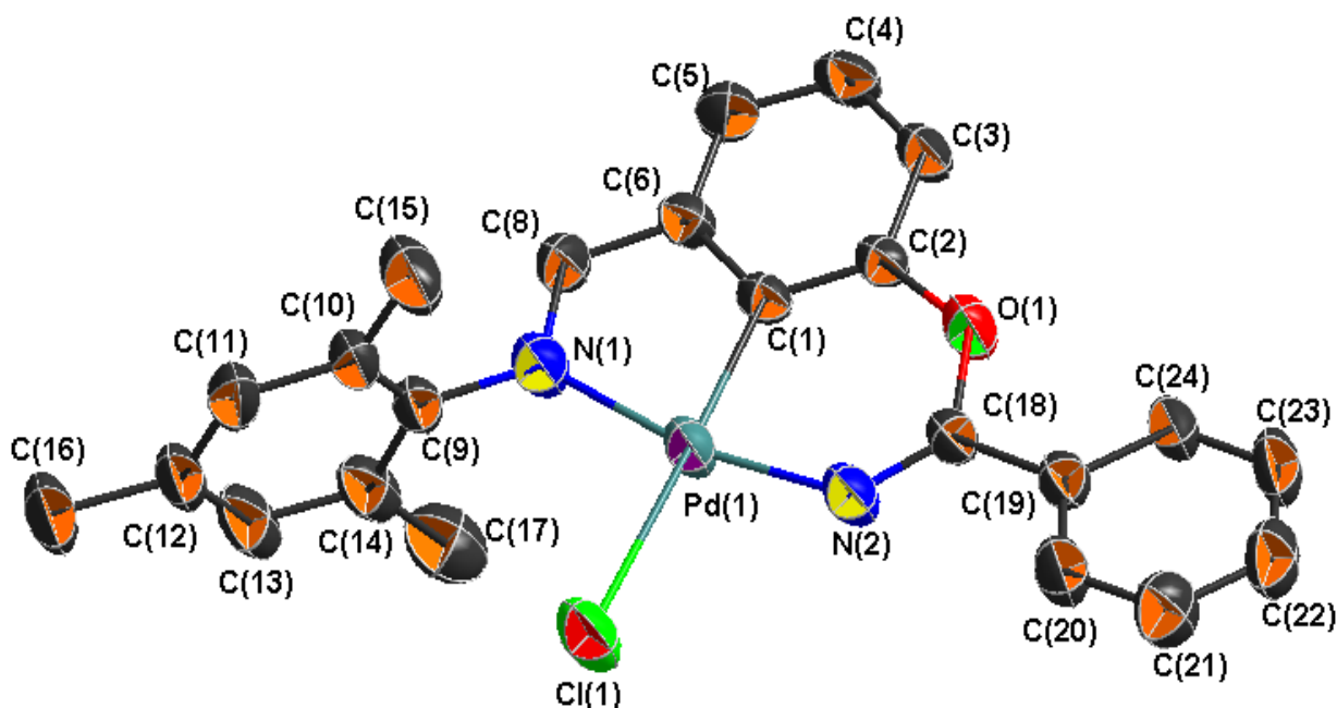
Figura 3.38. Estructura de difracción de rayos-X (Representación ORTEP al 40% de probabilidad) de una de las dos moléculas independientes del paladaciclos 3.7 . La mayoría de los átomos de hidrógenos y una molécula de cristalización ( \text{H}_2\text{O} ), se han omitidos para mayor claridad. Longitudes (Å) y ángulos (°) de enlaces seleccionados: Pd(1)–C(1) 1.938(4), Pd(1)–N(1) 2.049(4), Pd(1)–N(2) 1.993(4), Pd(1)–Cl(1) 2.410(14), O(1)–C(2) 1.403(6), O(1)–C(18) 1.337(6), C(18)–N(2) 1.284(6), C(6)–C(8) 1.441(7), C(8)–N(1) 1.284(6); C(1)–Pd(1)–Cl(1) 175.34(15), C(1)–Pd(1)–N(1) 80.88(18), C(1)–Pd(1)–N(2) 88.08(18), N(1)–Pd(1)–N(2) 168.71(15), N(1)–Pd(1)–Cl(1) 95.78(11), N(2)–Pd(1)–Cl(1) 95.38(12).
