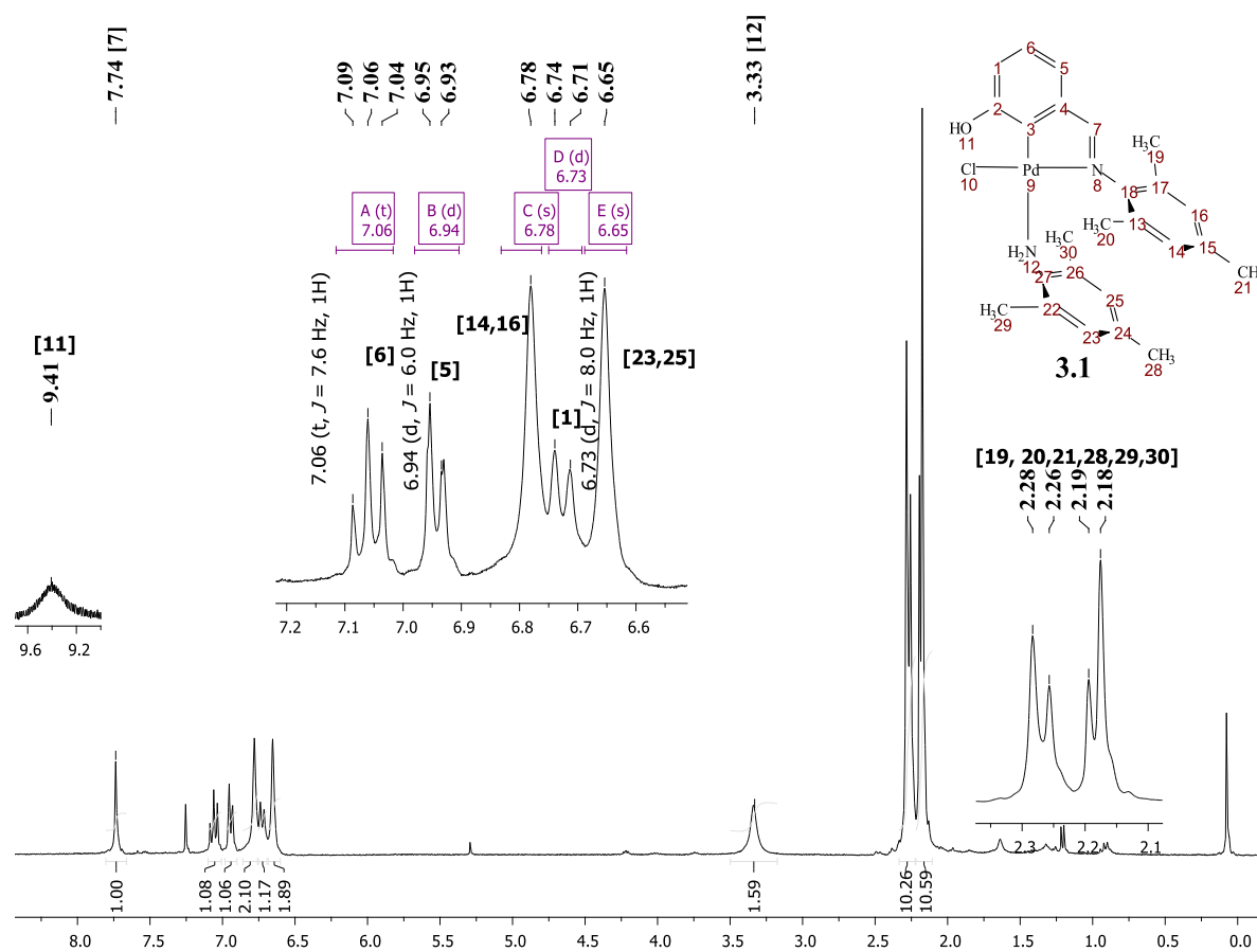
Figura 3.3. Espectro de RMN- ^1\text{H} (300 Hz, \text{CDCl}_3 ) del paladacilos monomérico 3.1.
