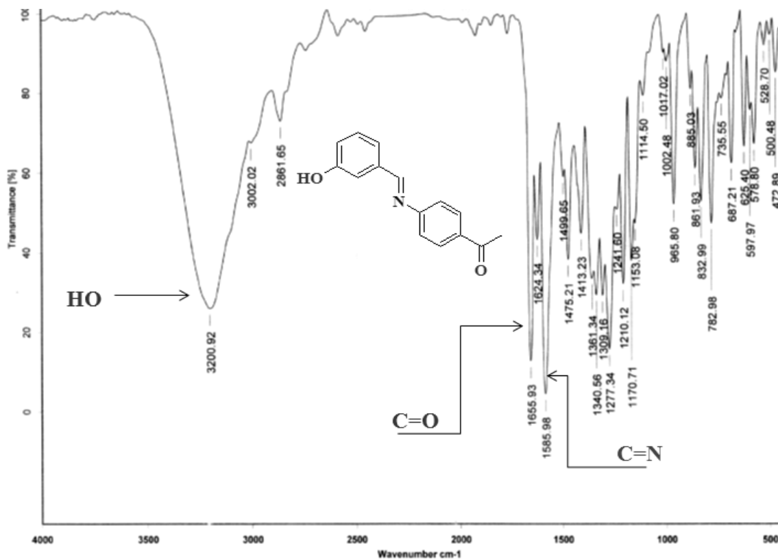
Figura 2.1. Espectro de IR del compuesto 2.12 y principales bandas de vibración.
