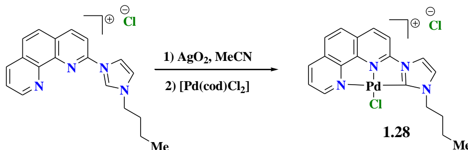
Esquema 1.9. Síntesis por transmetalación del paladaciclo carbénico 1.28 .
