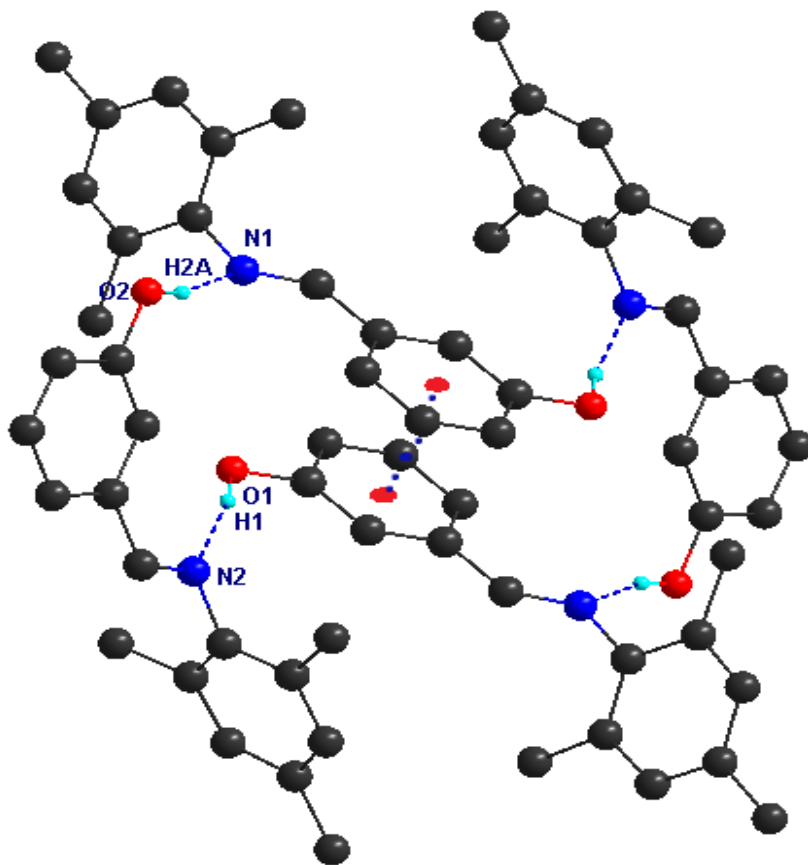
Figura 2.17. Tetrámero encontrado en el arreglo del compuesto 2.1 . Los átomos de hidrógeno que no intervienen en el arreglo son omitidos para mejor claridad.
