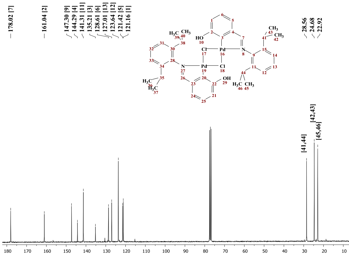
Figura 3.27. Espectro de RMN- ^{13}\text{C}\{^1\text{H}\} (75 MHz, \text{CDCl}_3 ) del compuesto paladado 3.5.
