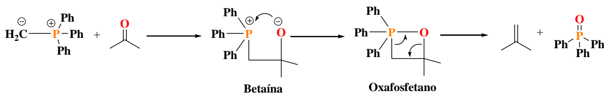
Esquema 3.14. Participación derivados orgánicos de fósforo en la formación de enlaces P-O.
