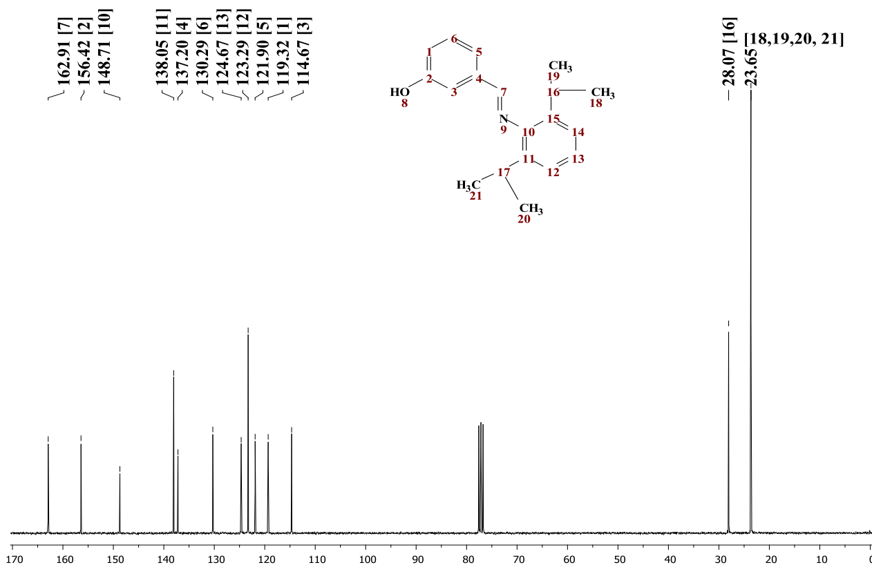
Figura 2.6. Espectro de RMN- ^{13}\text{C}\{^1\text{H}\} (75 MHz, \text{CDCl}_3 ) del compuesto 2.3 .
