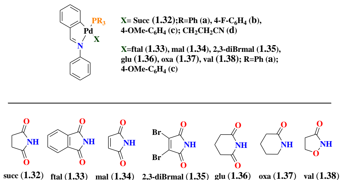
Figura 1.7. Paladaciclos monoméricos con ligantes fosfina e imidatos.
