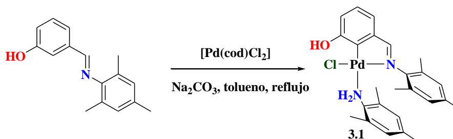
Esquema 3.1. Paladación del ligante imínico 2.1 y formación del complejo 3.1 .
