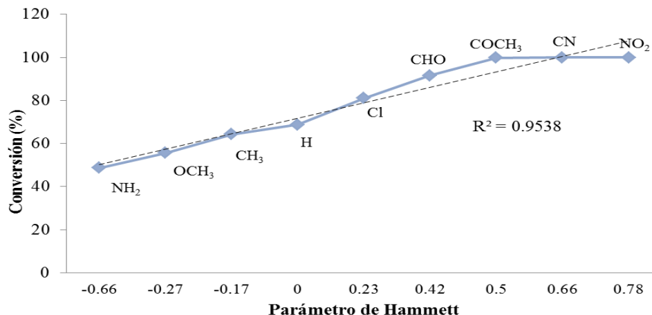
Gráfica 4.4. Conversión (%) en función del parámetro de Hammett ( \sigma ).
