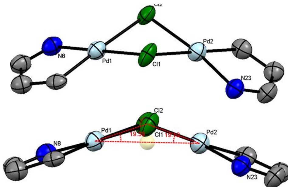
Figura 3.35. Representación ( MERCURY ) de la estructura parcial del complejo 3.6 , exhibiendo ausencia de coplanaridad entre los centros metálicos de paladio y sus ambientes de coordinación con ángulo desviación \alpha de 19.12 y 19.39°.
