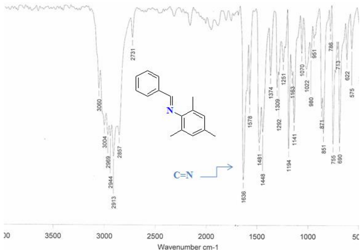
Figura 2.25. Espectro de IR del compuesto imínico deshidroxilado 2.14 .
