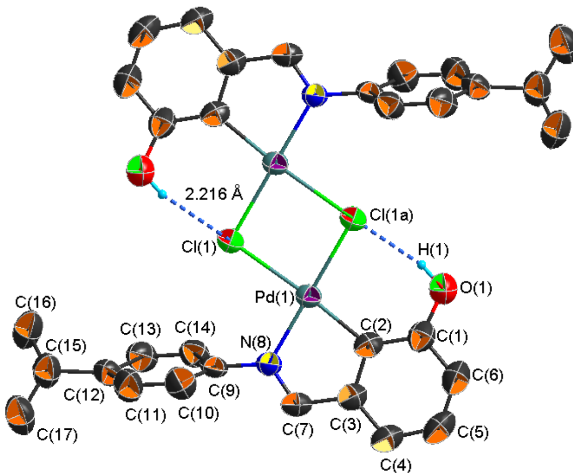
Figura 3.15. Representación (ORTEP al 50% de probabilidad) del estructura cristalina polimórfica con el grupo espacial P2_1/c del paladacillo dimérico 3.3 , exhibiendo dos interacciones intramoleculares de enlaces de hidrógeno O-H---Cl. La mayoría de los átomos de hidrógenos, se han omitidos para mayor claridad. Longitudes (Å) y ángulos (°) de enlaces seleccionados: Pd(1)-C(2) 1.995(5), Pd(1)-N(8) 2.029(4), Pd(1)-Cl(1) 2.46(1), Pd(1)-Cl(1)a 2.335(1), C(7)-N(8) 1.281(6); C(2)-Pd(1)-N(8) 80.78(2), C(2)-Pd(1)-Cl(1) 175.88(1), C(2)-Pd(1)-Cl(1)a 99.16(1), N(8)-Pd(1)-Cl(1) 95.10(1), N(8)-Pd(1)-Cl(1)a 175.18(1), Cl(1)-Pd(1)-Cl(1)a 84.93(4).
