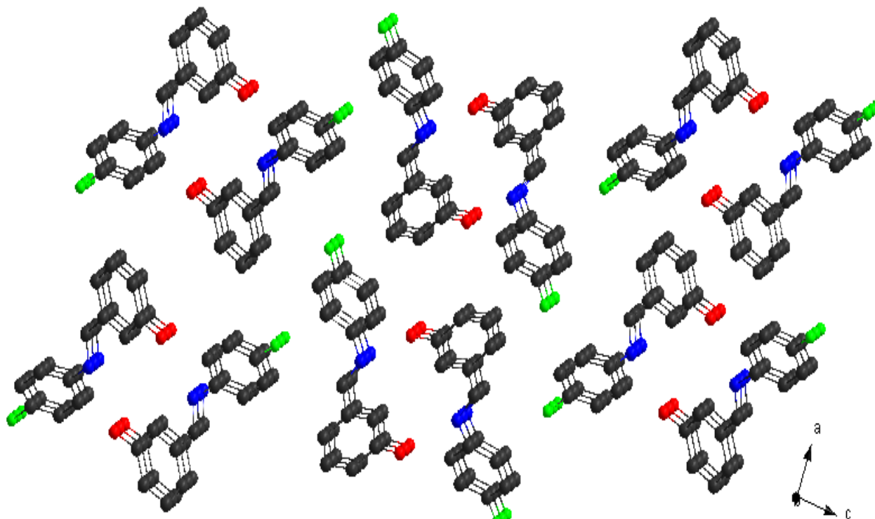
Figura 2.24. Arreglo en las tres dimensiones del compuesto 2.11 , los átomos de hidrógeno son omitidos para una mejor claridad.
