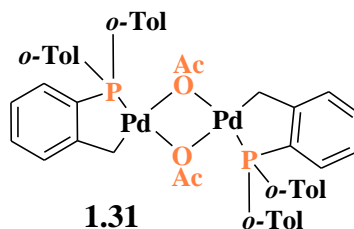
Figura 1.6. Paladaciclo de trio- o -tolilfosfina o de Hermann-Beller.
