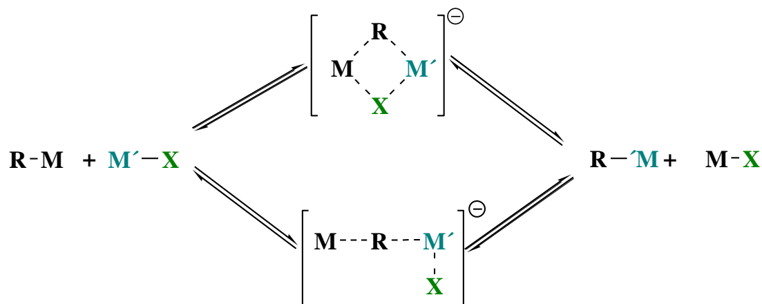
Esquema 1.6. Proceso de transmetalación.
