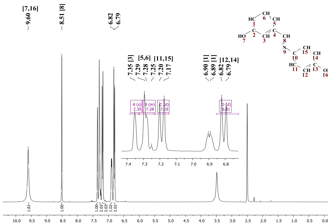
Figura 2.7. Espectro de RMN- 1 H (300 MHz, DMSO- d 6 ) del compuesto 2.7 .
