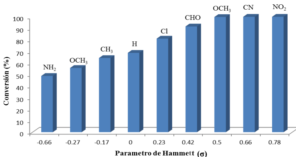
Gráfica 4.3. Conversión (%) de la reacción de Suzuki-Miyaura empleando el complejo 3.5 .
