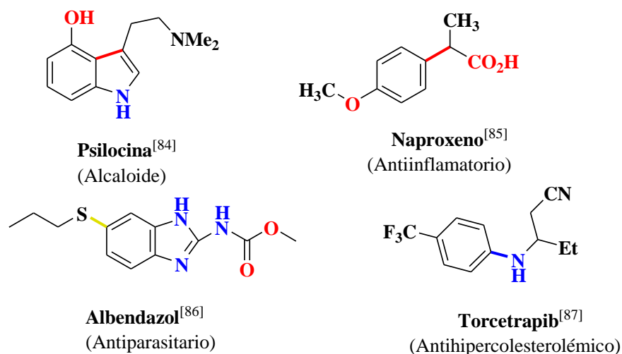
Figura 4.1. Compuestos importantes que presentan enlaces C-C y C-heteoátomo.
