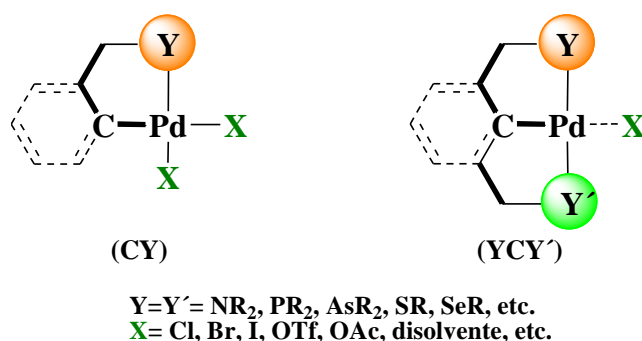
Figura 1.1. Clasificación de los paladaciclos de acuerdo al fragmento orgánico.
