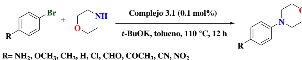
Esquema 4.5. Reacción de acoplamiento cruzado C-N catalizada por el complejo 3.1 .
