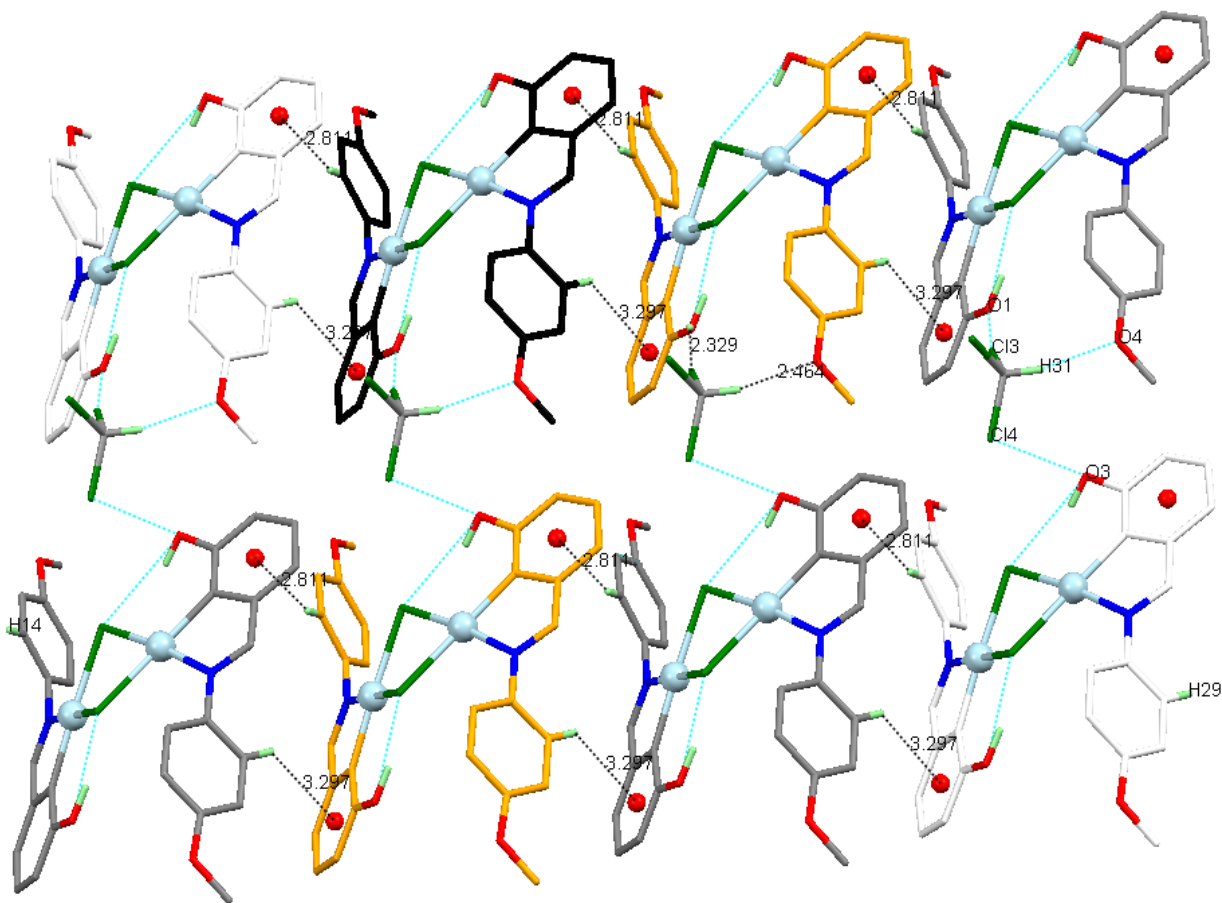
Figura 3.34. Fragmento del arreglo cristalino del complejo de paladio 3.6 (Representación MERCURY), mostrando interacciones de tipo C-H... \pi a lo largo del eje a , así como asociaciones de enlaces de hidrógeno (OH...Cl y C-H...O) con las moléculas de cloroformo. Para mayor claridad se ha omitido el desorden de los átomos de cloro. Únicamente se muestran los átomos de hidrógeno que participan en las interacciones.
