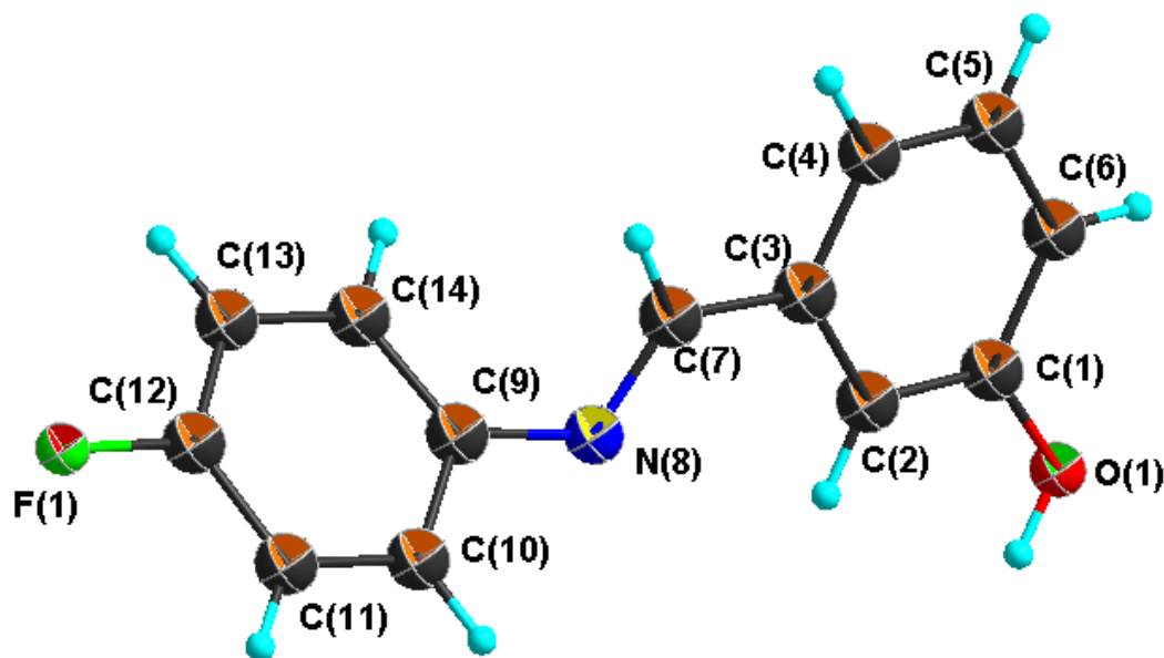
Figura.2.15. Estructura molecular de una las dos moléculas independientes del ligante 2.11 con elipsoides al 50% de probabilidad. Longitudes de enlaces seleccionados (Å) y ángulos (°): C(7)-N(8) 1.268(4), C(3)-C(7) 1.457(5), C(2)-C(3) 1.389(5), C(1)-O(1) 1.350(4), C(1)-C(2) 1.382(5), C(1)-O(1) 1.350(4), C(9)-N(8) 1.427(4), C(9)-C(10) 1.389(5), C(12)-F(1) 1.366(4); N(8)-C(7)-C(3) 125.7(3), C(7)-N(8)-C(9) 118.1(3), O(1)-C(1)-C(2) 123.5(3), F(1)-C(12)-C(11) 117.9(3).
