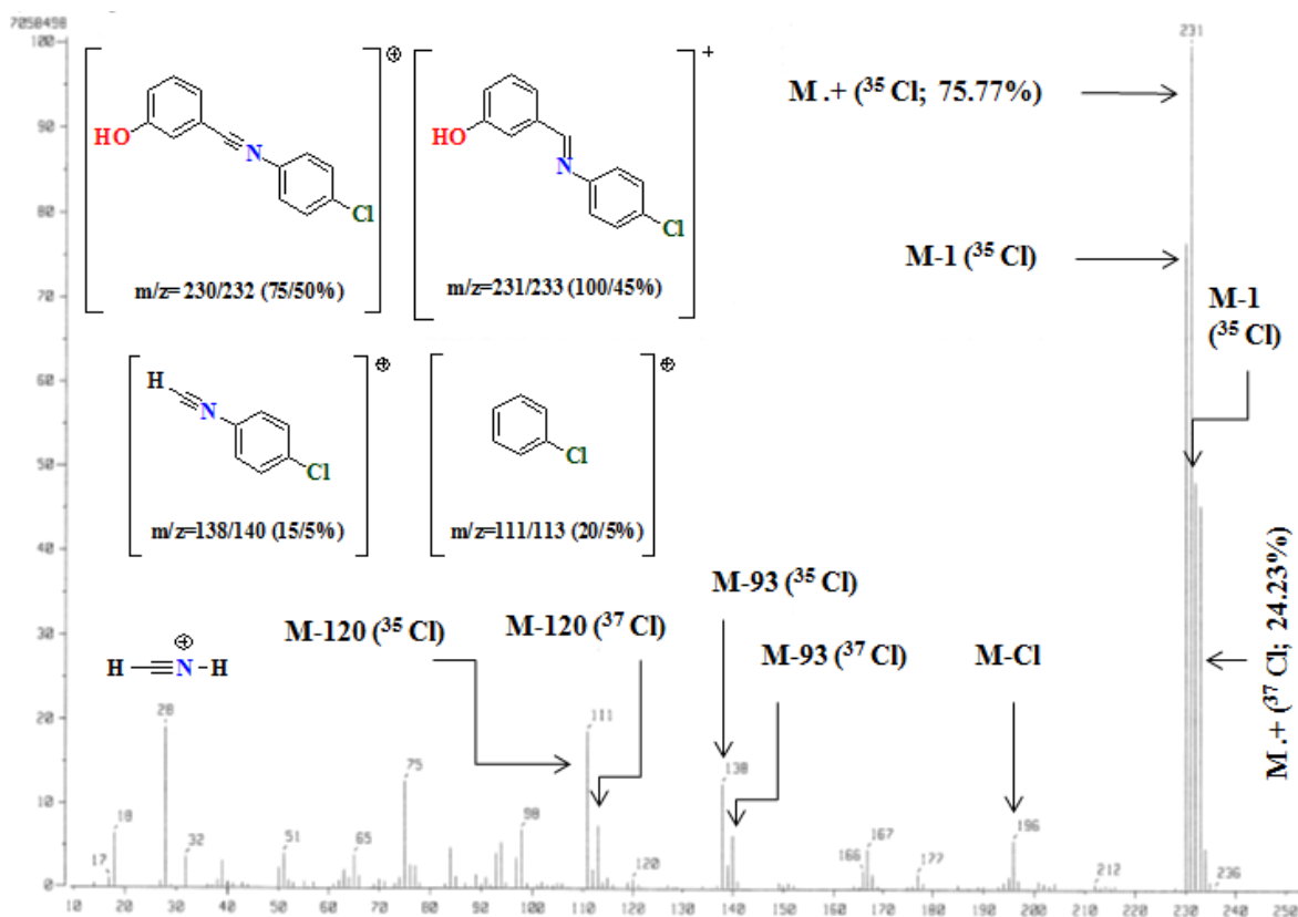
Figura 2.2. Espectro de masas del ligante 2.10 y principales fragmentos con abundancias isotópicas conocidas.
