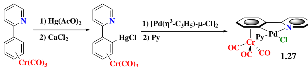
Esquema 1.8. Obtención del paladaciclo monomérico quiral 1.27 por transmetalación.
