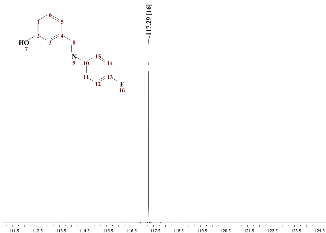
Figura 2.11. Espectro de RMN- ^{19}\text{F} (282 MHz, \text{CDCl}_3 ) del compuesto 2.11 .
