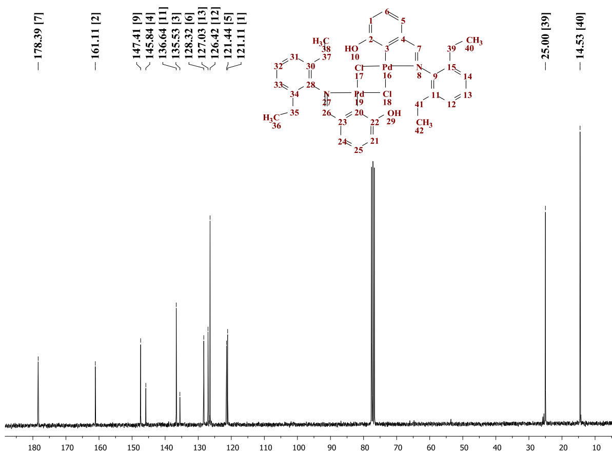
Figura 3.22. Espectro de RMN- ^{13}\text{C}\{^1\text{H}\} (75 MHz, \text{CDCl}_3 ) del compuesto paladado 3.4 .
