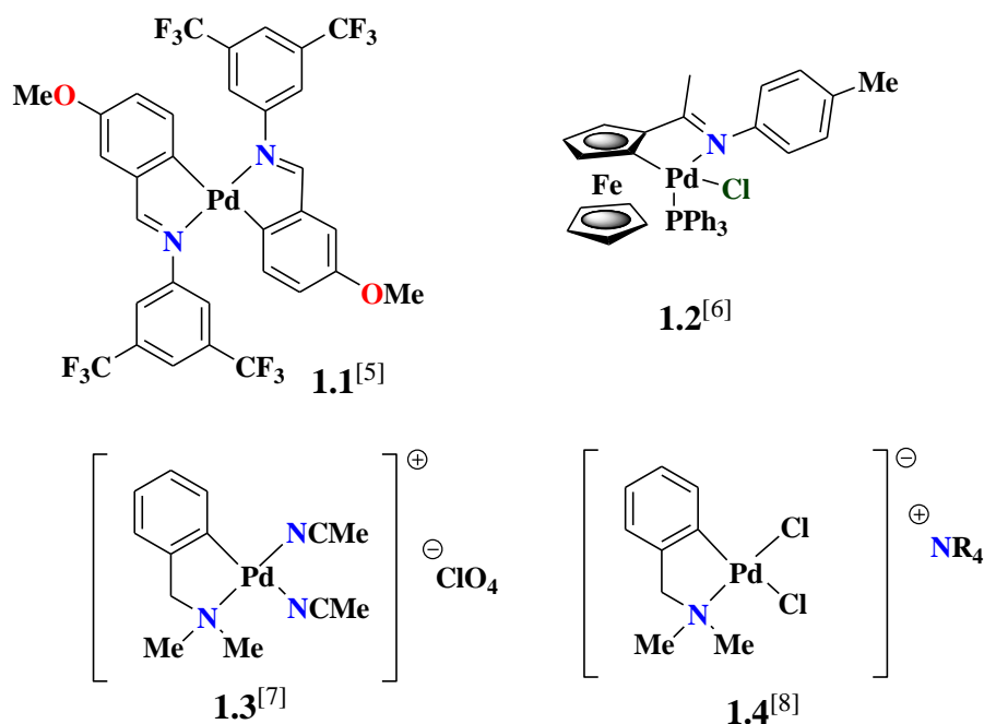
Figura 1.3. Diferentes tipos de paladacilos CY .
