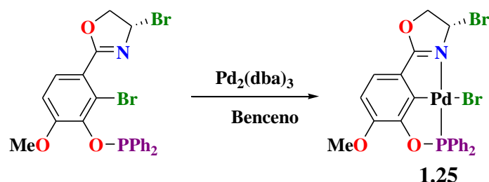
Esquema 1.5. Obtención del paladaciclo PCN a través de una adición oxidativa.
