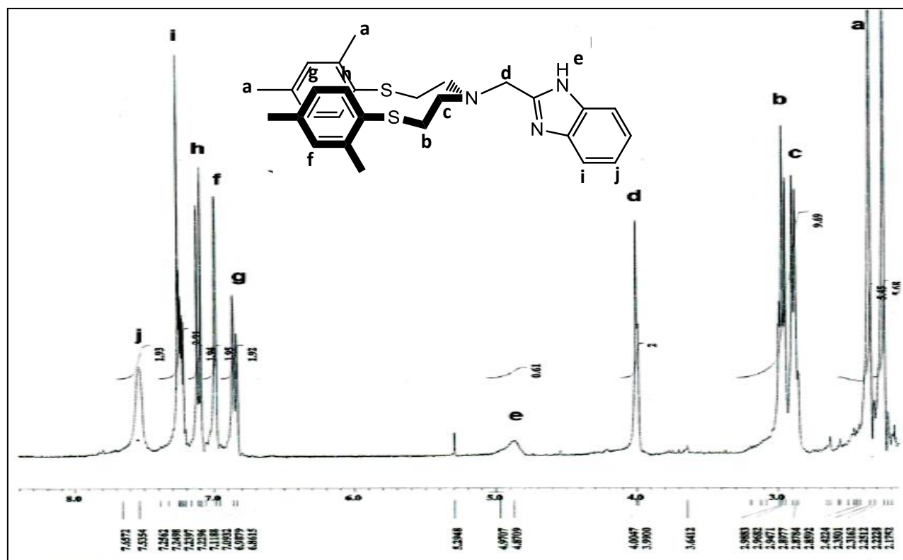
Figura 15. Espectro de RMN ^1\text{H} de L2 en \text{CDCl}_3 .
