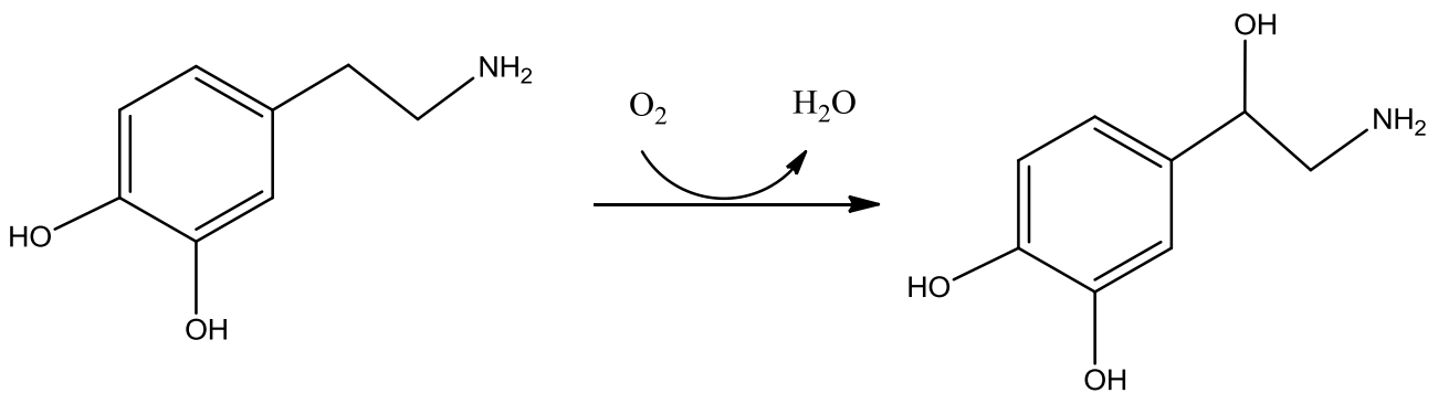
Esquema 1. Reacción catalizada por D \beta M.
