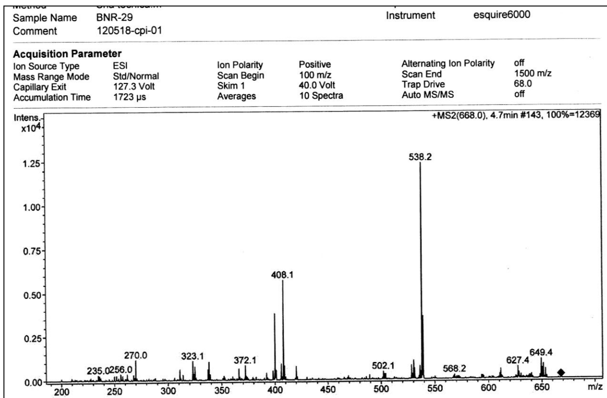
Figura 32. Espectro de masas ESI de [CuL 2 ]PF 6 .
