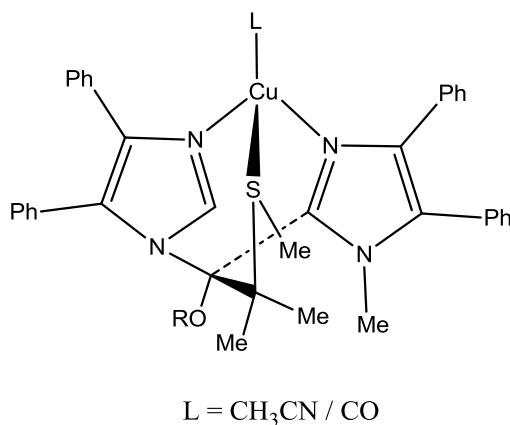
Figura 11. Ligante tripodal sintetizado por Zhou y Nicholas.
