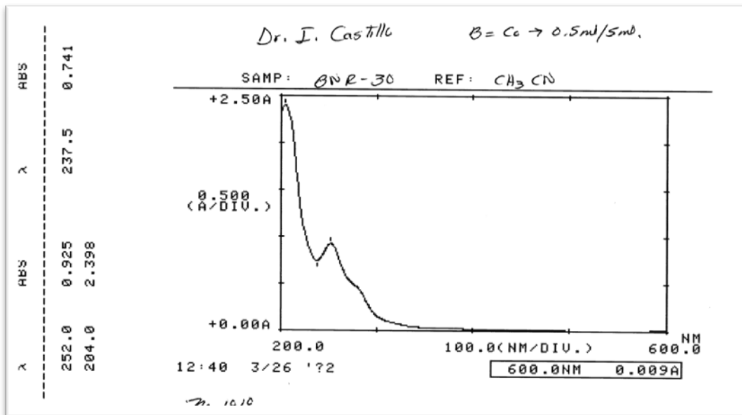
Figura 36. Espectro UV-vis de [CuL_3](AcO)_2 .
