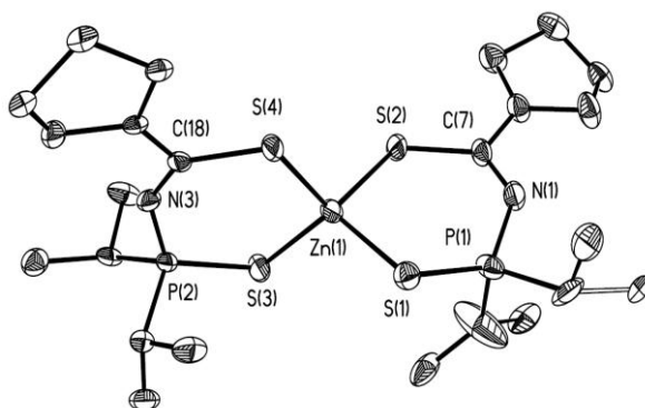
Fig. 5.2: Estructura molecular del compuesto de coordinación \text{Zn}\{\eta^2\text{-S,S-}[P(1)C(7)N(1)C(S)NC(S)NC_4H_8]\}_2 (ZnSS).
