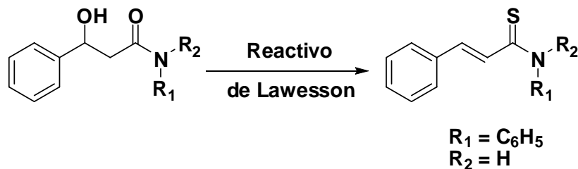
Esquema 3.14. Reactividad de ω-hidroxi amidas frente al reactivo de Lawesson.
