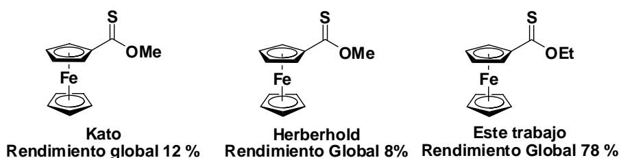
Esquema 2.16. Síntesis de ferroceniltionioéster vía carbenos de Fischer.
