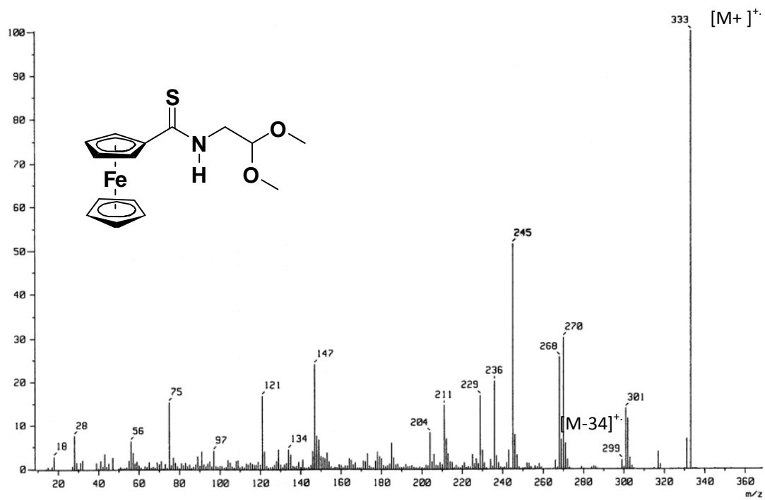
Espectro 3.11. Espectro de Masas para el compuesto 18 en ( IE^+ ).
