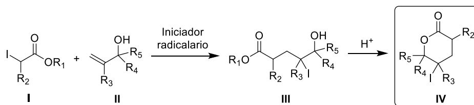
Esquema 18. Propuesta sintética.
