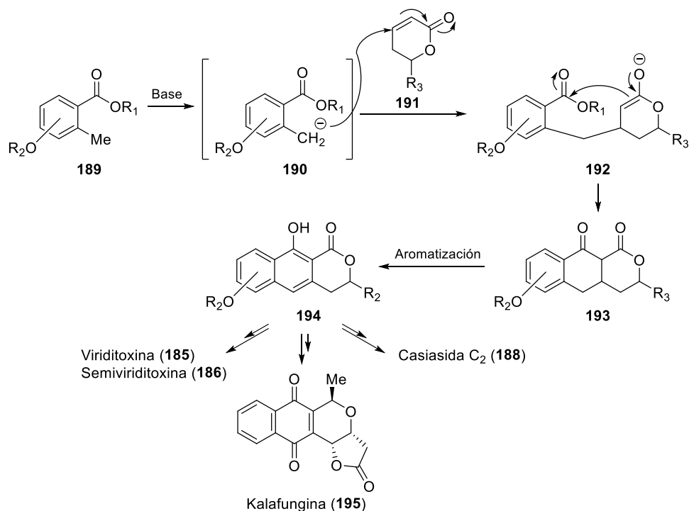
Esquema 35. Mecanismo y aplicaciones de la ciclación de Staunton-Weinreb.
