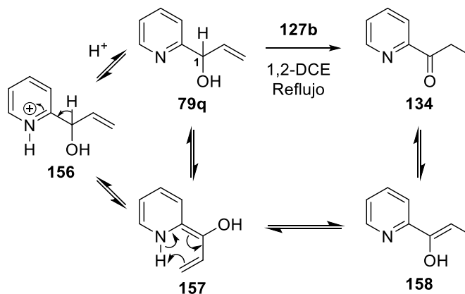
Esquema 27. Mecanismo reportado para la generación de 134 .
