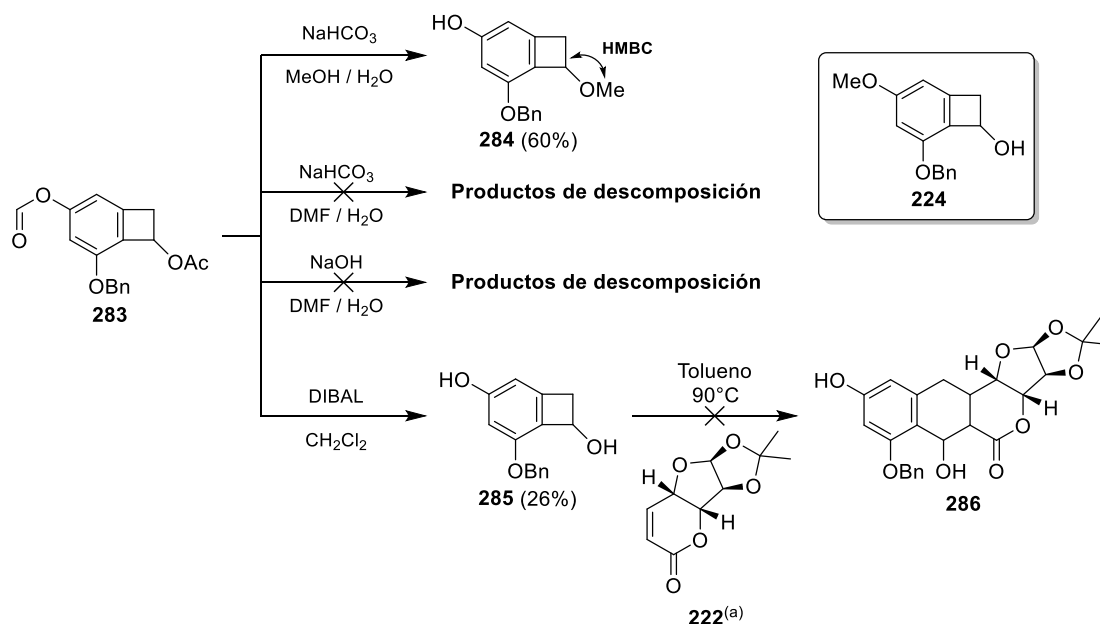
Esquema 50. Hidrólisis del formiato 283 y ensayo de reacción Diels-Alder.
