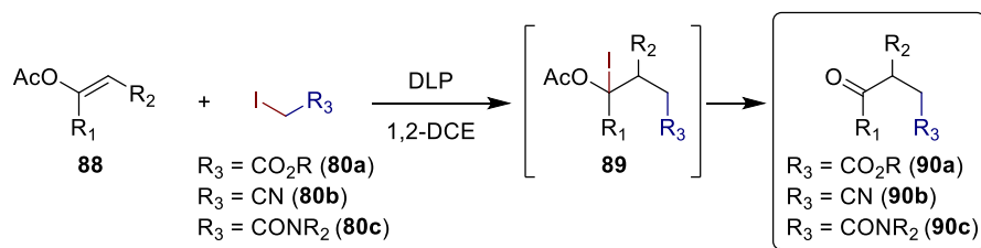
Esquema 16. Secuencia para la obtención de compuestos 1,4-dicarbonilo (90).
