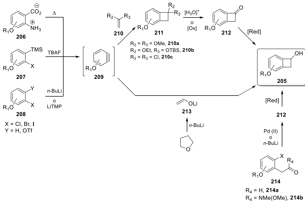
Esquema 37. Métodos comunes para la preparación de benzociclobutenos ( 205 ).
